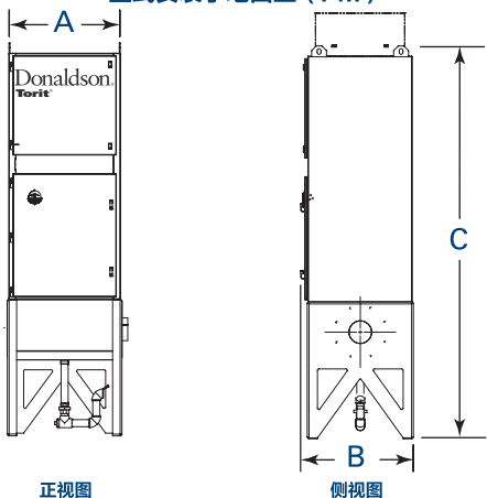
WSO 20, 25-1 立式安装于地面上 (FM)
