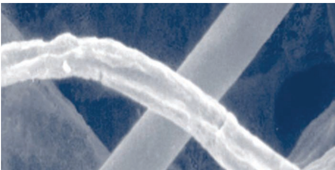
Handelsübliche Filtermedien (600px) – Konventionelle Filtermedien haben einen Abstand von bis zu 60 µm zwischen den Fasern, wodurch der Staub tief in das Filtermedium eindringen kann.
