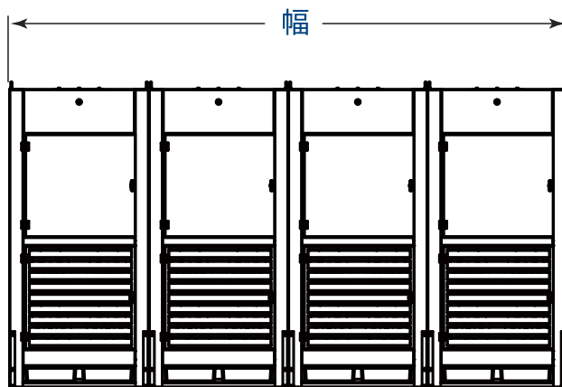
正面図 DWST 4-4, DWST 6-4
