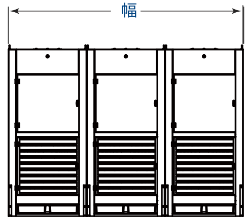
正面図 DWST 4-3, DWST 6-3
