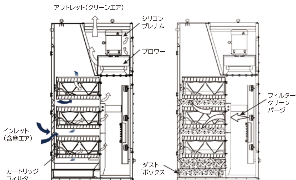
通常運転時フロー
