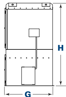
Right Side View UMA 450-750 (750 Shown)
